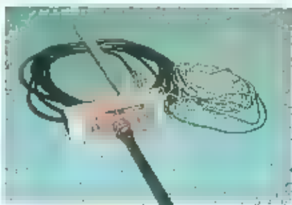
Een zelfgemaakte isolator van plexiglas waarop een spriet uit de dump is geschroefd. De gemonteerde grondpen maakt het mogelijk de spriet stevig in de grond te plaatsen waarna de radialen kunnen worden uitgerold.
